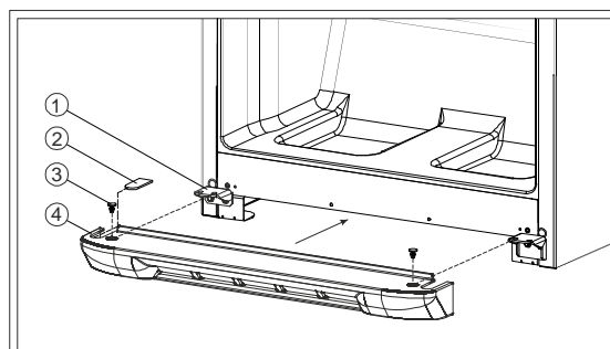
Схема установки нижней декоративной накладки (дверь холодильника условно не показана)
